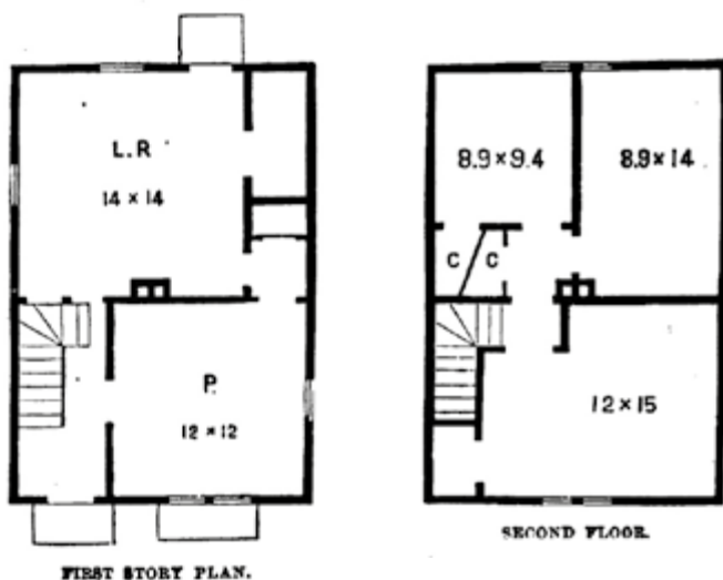
51. Plan type d'une maison d'un étage et demi, tiré du modèle n°VIII de Village and farm cottages de Cleaveland, Backus and Backus publié en 1869.
