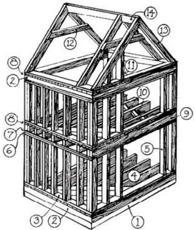
45. Dessin schématique d'une structure de type « plateforme ».
